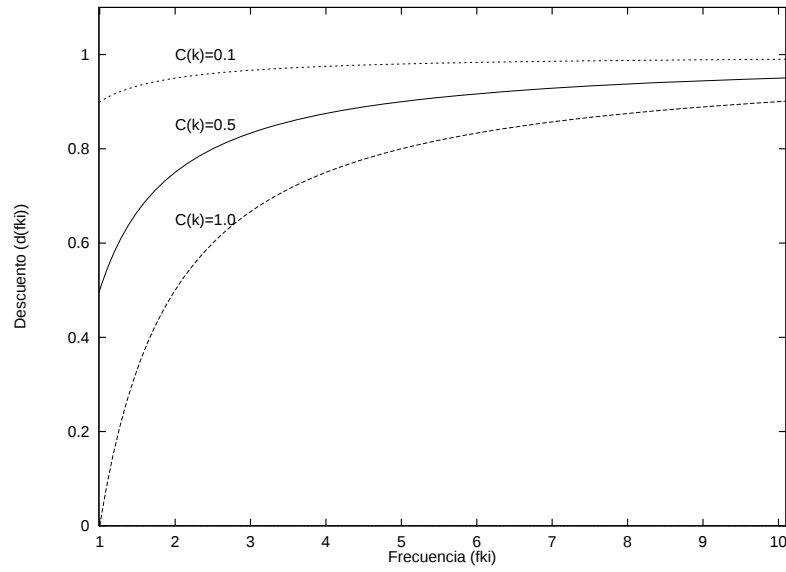
Figura 4.5: Comportamiento de la función de descuento en función de la frecuencia (BDFF) considerando distintos valores de C(k) .
